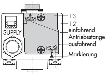
Bild 5 · Direktanbau – Stelldruckanschluss für Antrieb Typ 3277 mit 240, 350 und 700 cm 2
